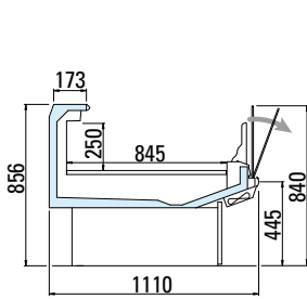
VDB MAXI SELF
